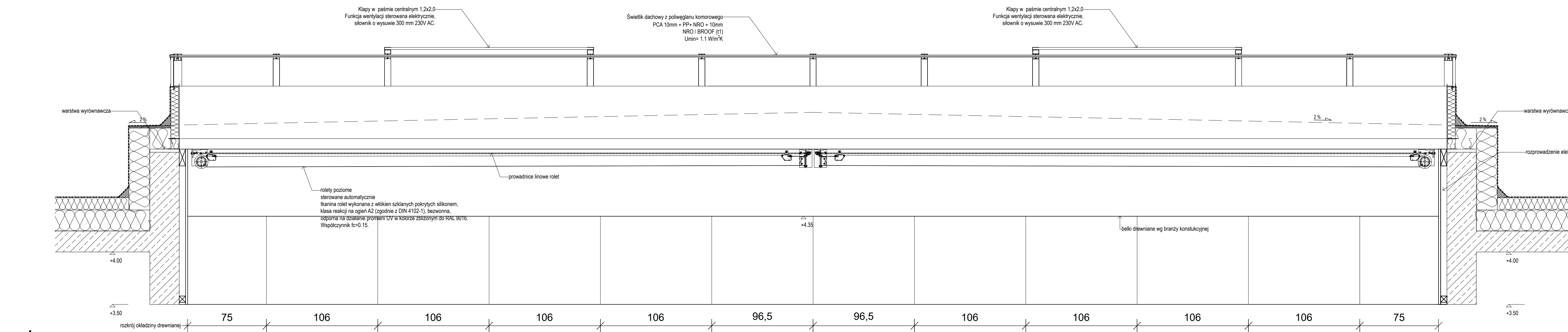
Detal 5 - przekrój 2-2, 1:20
