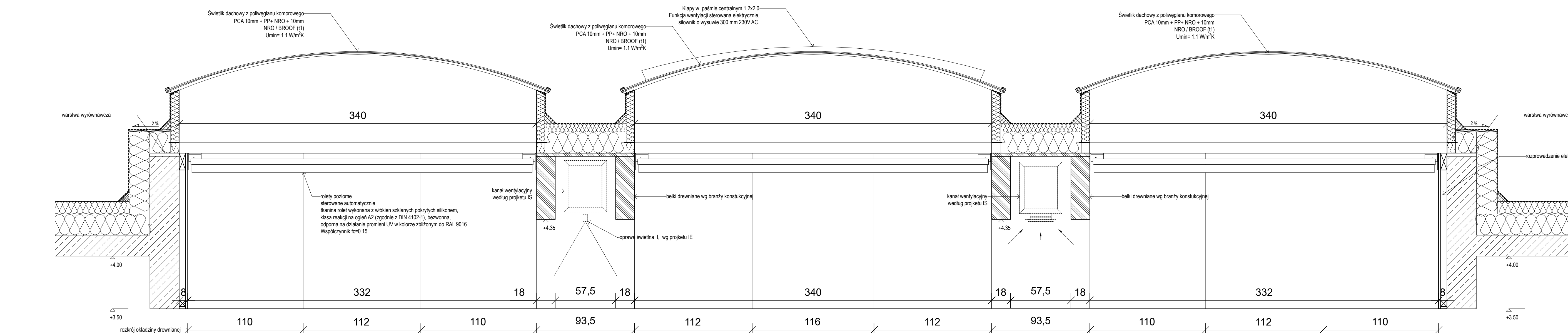
Detal 5 - przekrój 2-2, 1:20
