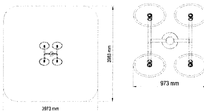
Strefa bezpieczeństwa dla urządzenia ST-007
